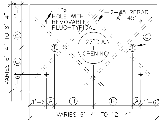
LID PLAN
